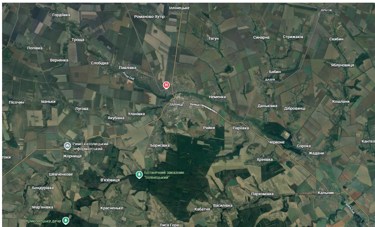
Рисунок 3.3. Картосхема лісів на території Іллінецької громади
