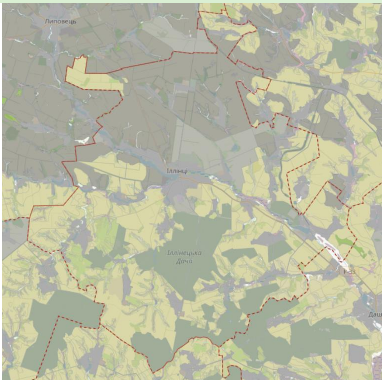
Рисунок 3.2. Види ґрунтів на території Іллінецької громади
