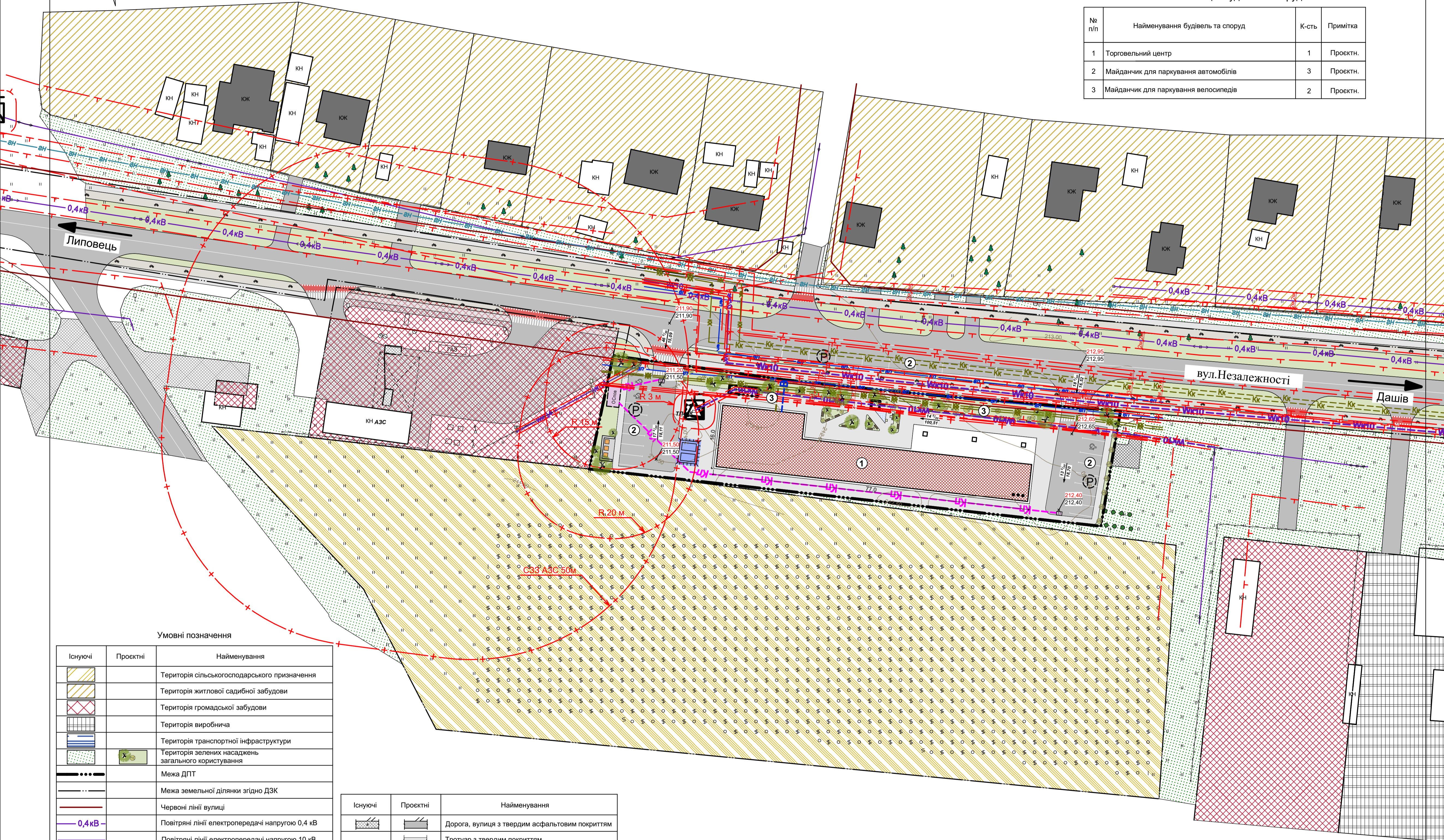
Умовні позначення до вертикального планування
